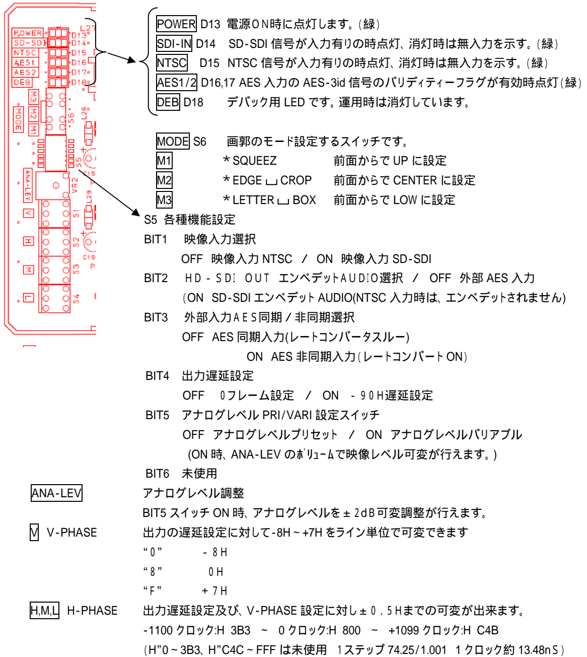
図 2 背面視
